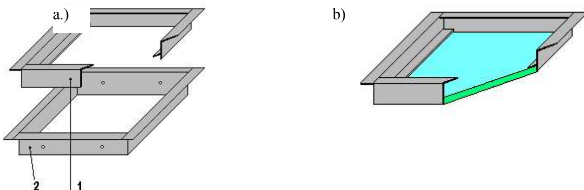
Rys. 1. A) 1 – część ruchoma klap, 2 – część stała, konstrukcja nośna klap. B) część ruchoma klap, po wypełnieniu płytą gipsową.
